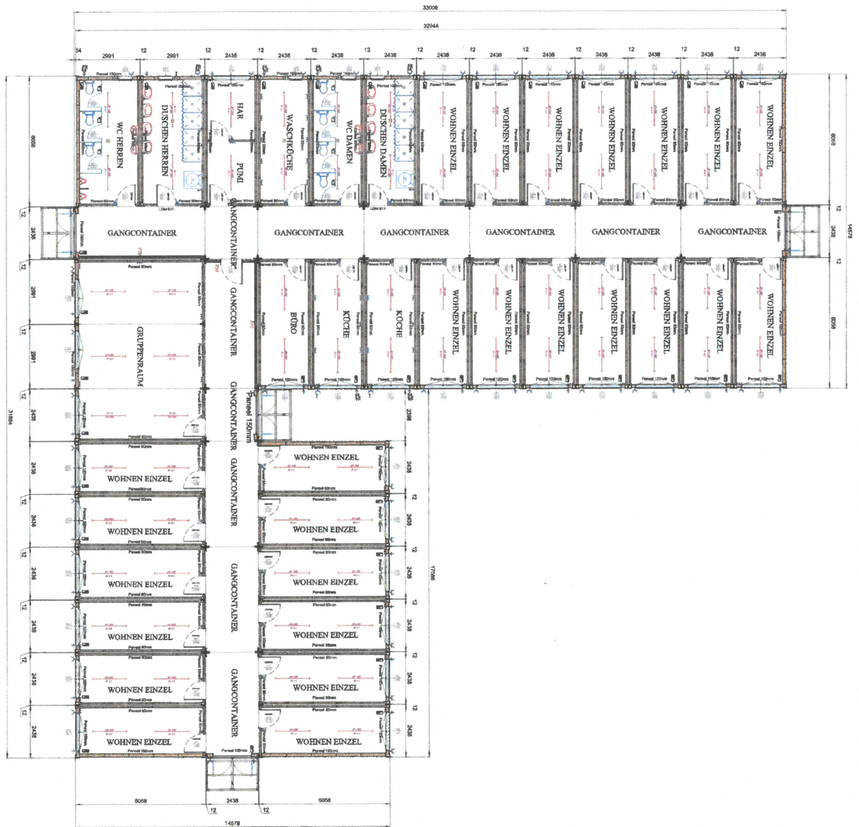
Grundriss Containereinheit (L-Container)
